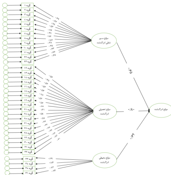
شکل ۲. نتایج تحلیل عاملی برای مدل تک عاملی مرتبه دوم. اعداد، ضریب رگرسیونی استاندارد شده
