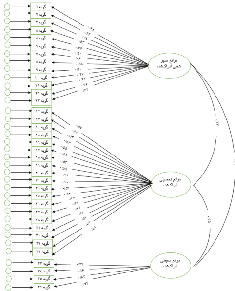
شکل ۱. نتایج تحلیل عاملی برای ساختار سه عاملی مرتبه اول. اعداد، ضریب رگرسیونی
